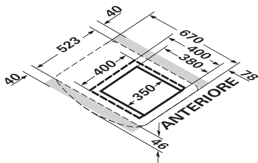
Fig. 11 - distributore d'aria
