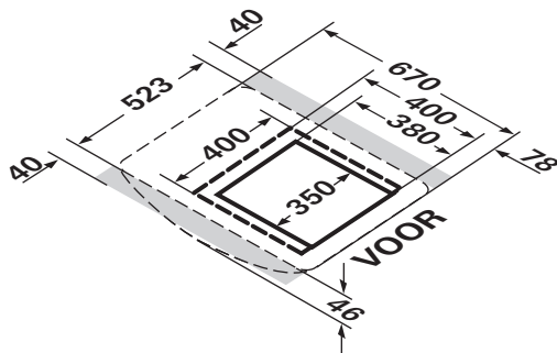
Afbeelding 11 – Luchtverdeler
