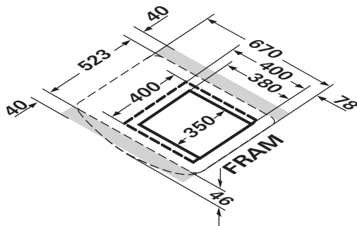
Bild 11 – luftspredare
