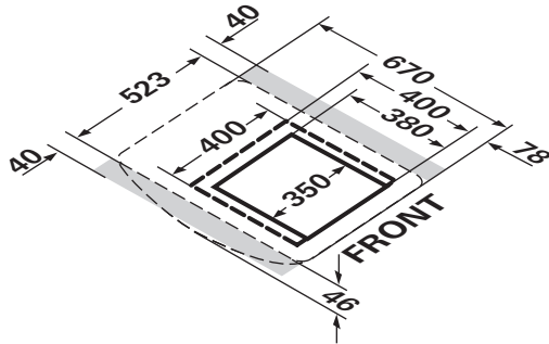
Bild 11 - Luftverteiler
