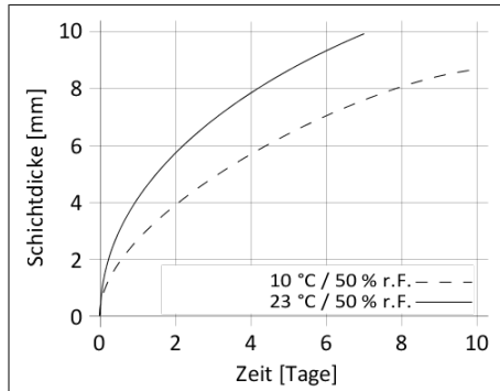
Diagramm 1: Durchhärtengeschwindigkeit SikaTack® DRIVE (Purform®)
