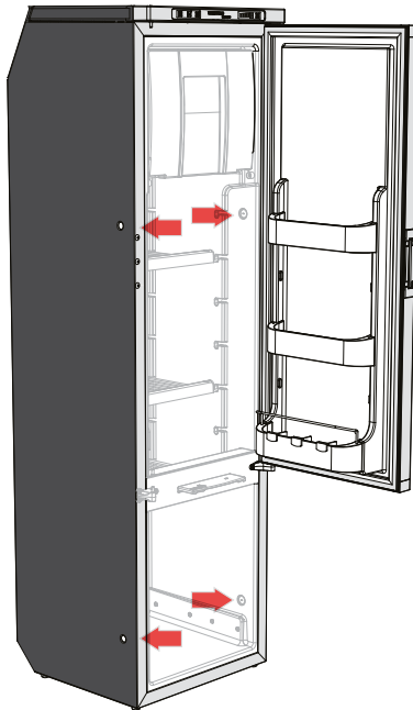
FIG.1 - FISSAGGI INTERNI A SCOMPARSA INTERNAL CONCEALED FIXING
